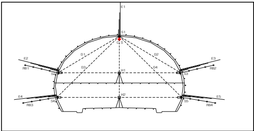
▶ 지보패턴 : TYPE 4
