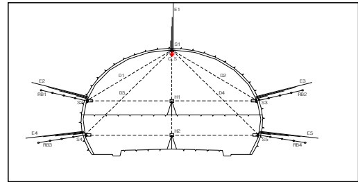
▶ 지보패턴 : TYPE 4
